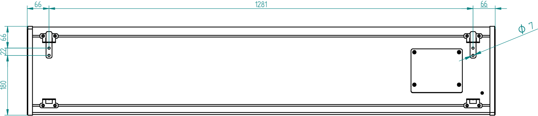
Vista trasera
