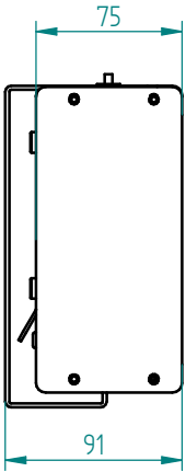
Vista lateral
