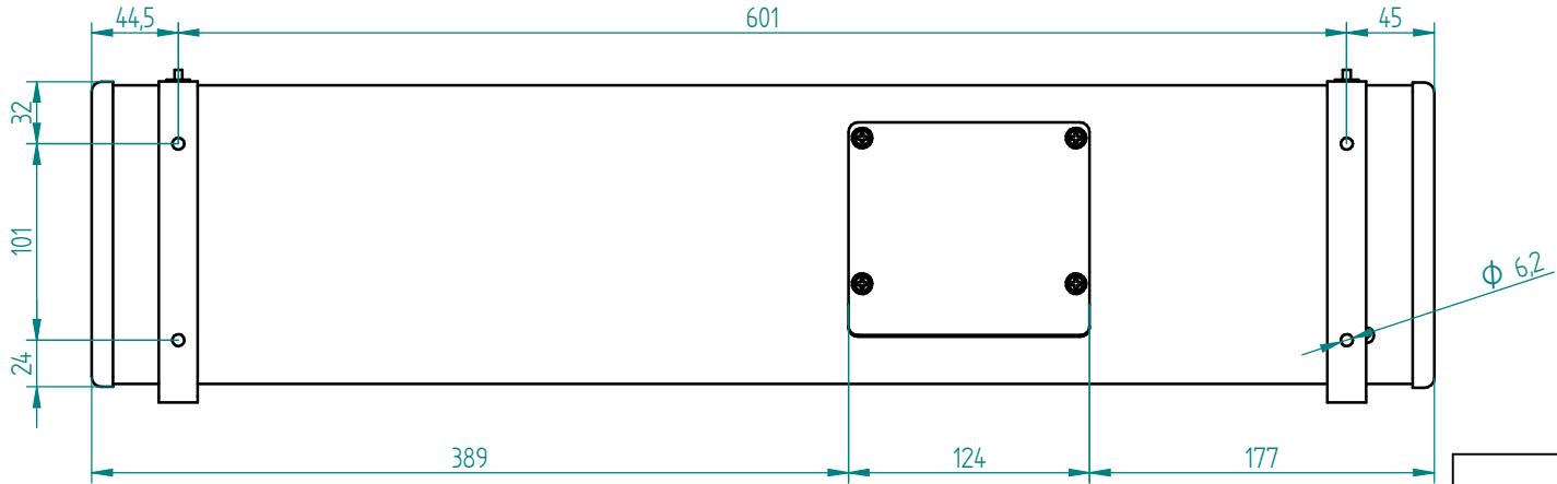
Vista trasera
