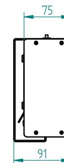
Vista lateral
