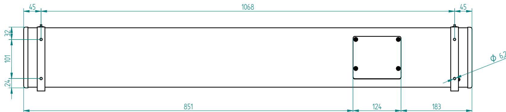
Vista trasera
