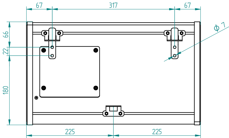
Vista trasera
