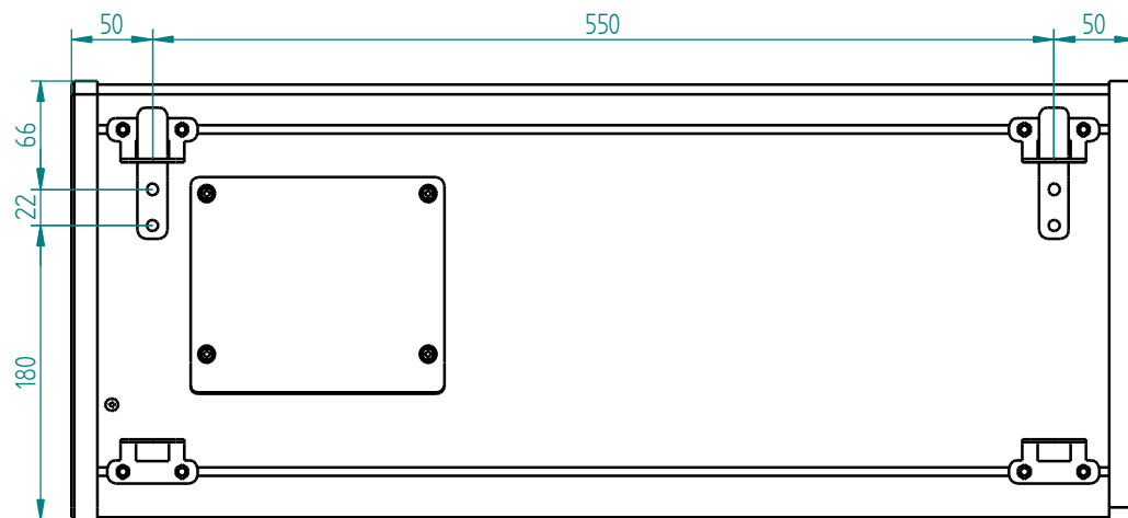
Vista trasera
