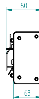
Vista lateral
