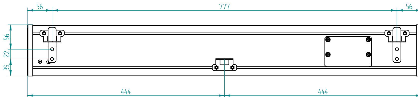
Vista trasera
