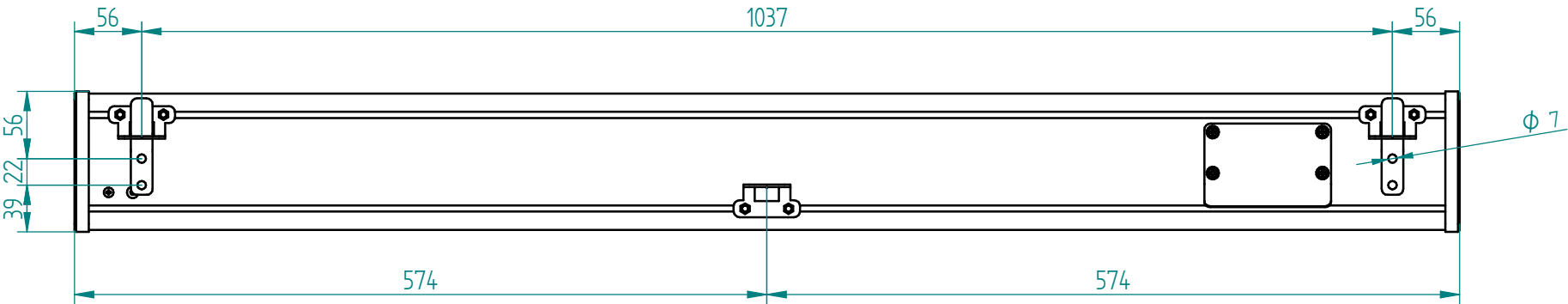
Vista trasera
