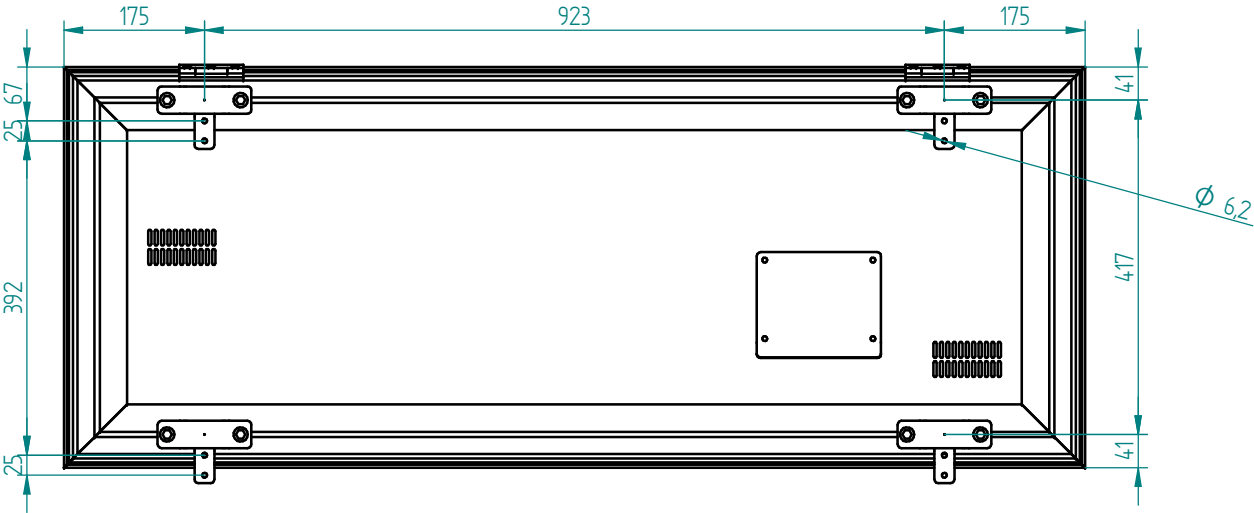
Vista trasera
