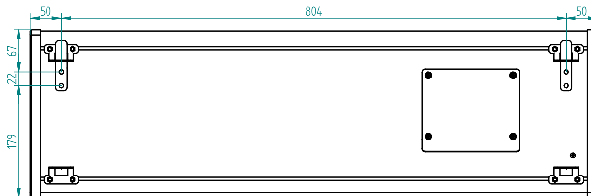
Vista trasera
