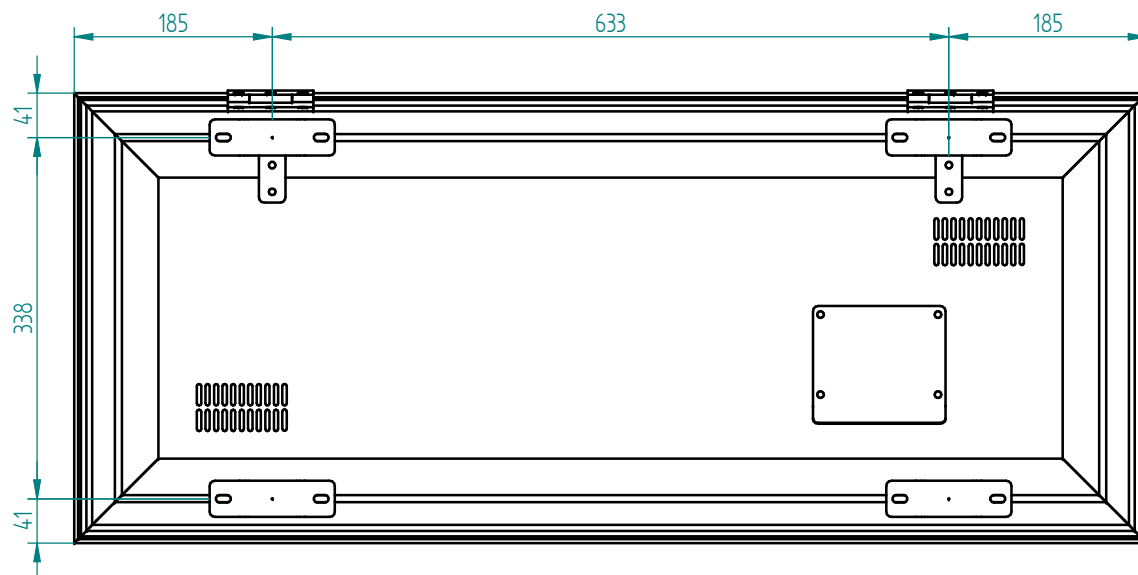
Vista trasera
