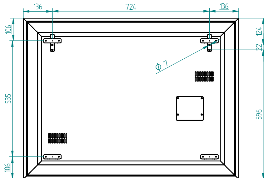
Vista trasera
