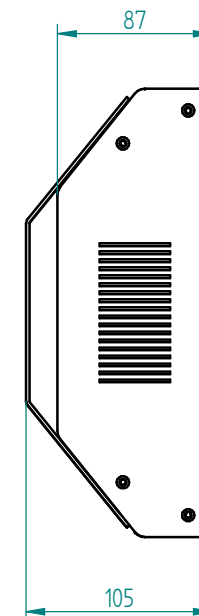
Vista lateral
