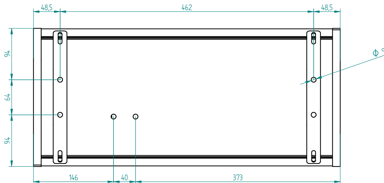
Vista trasera
