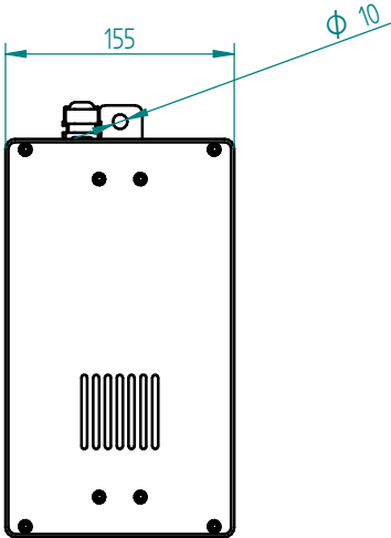
Vista lateral
