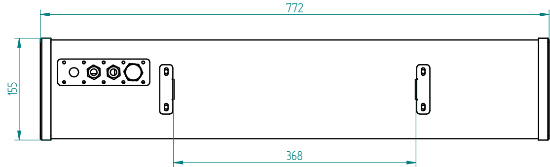
Vista superior
