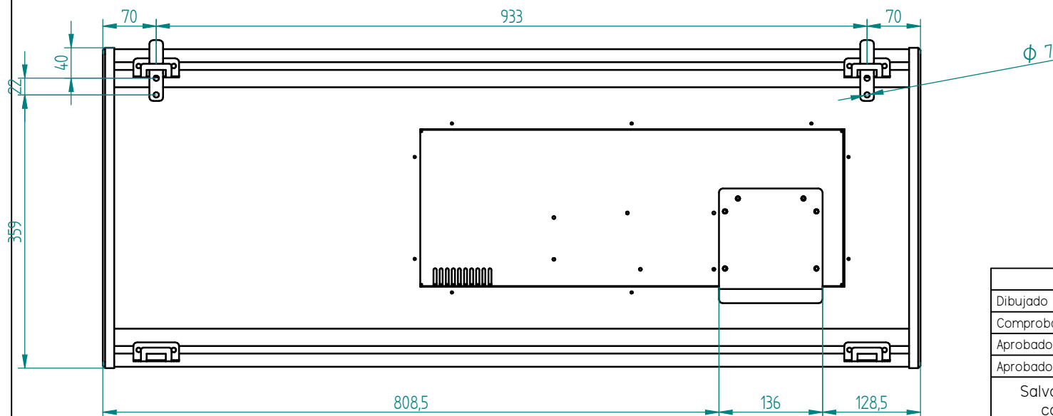
Vista trasera
