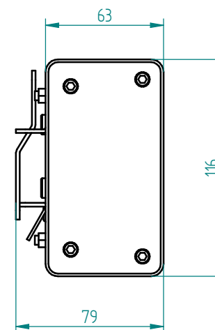
Vista lateral
