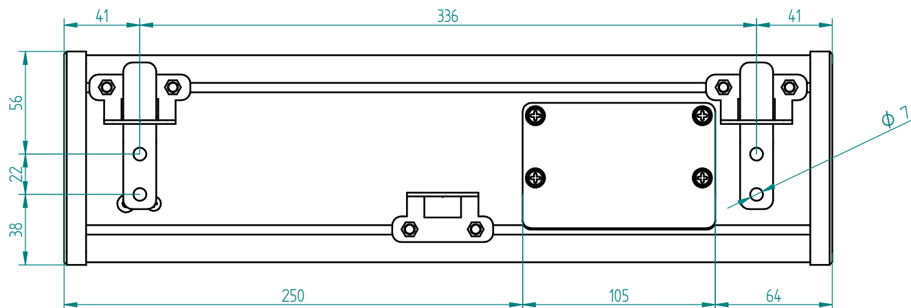
Vista trasera
