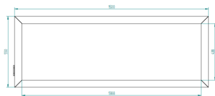
MGM2A CABECERA 550
