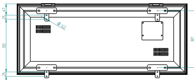
Vista trasera
