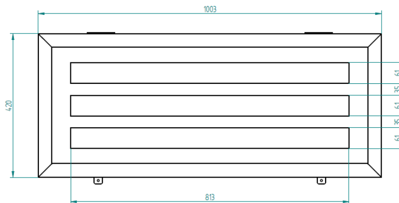
Vista trasera
